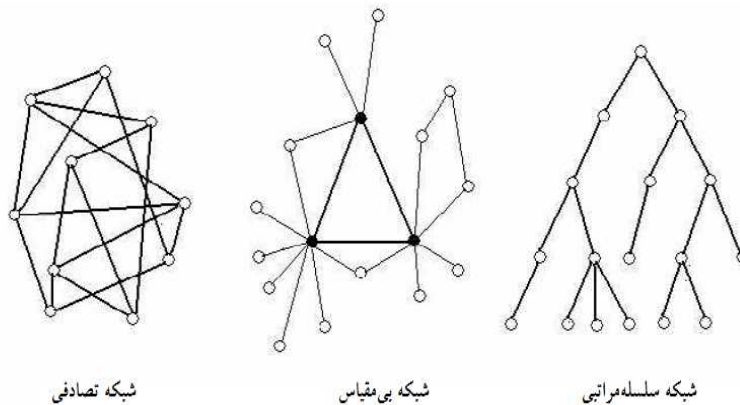
شکل ۱. انواع شبکه
